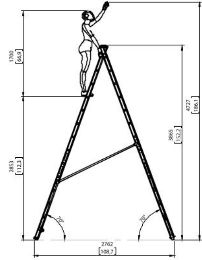
Teknik Çizim Technical Drawing
