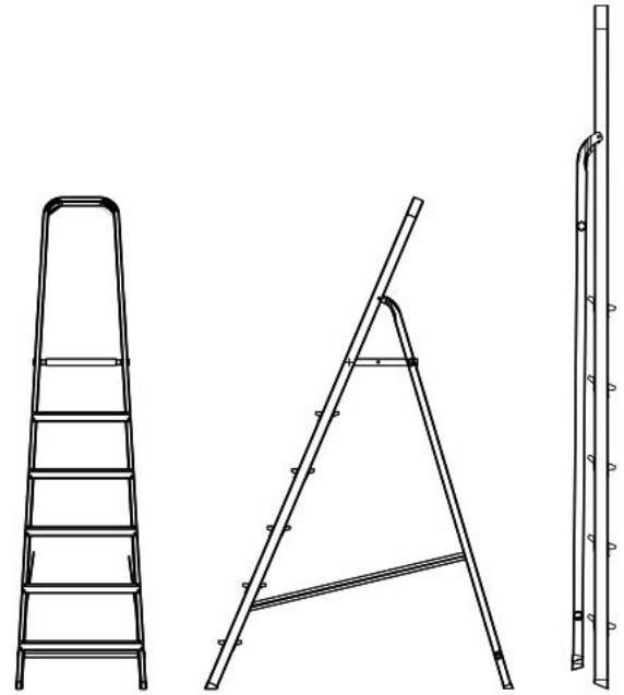
Teknik Çizim Technical Drawing
