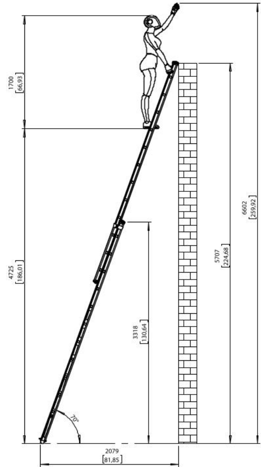
Teknik Çizim Technical Drawing
